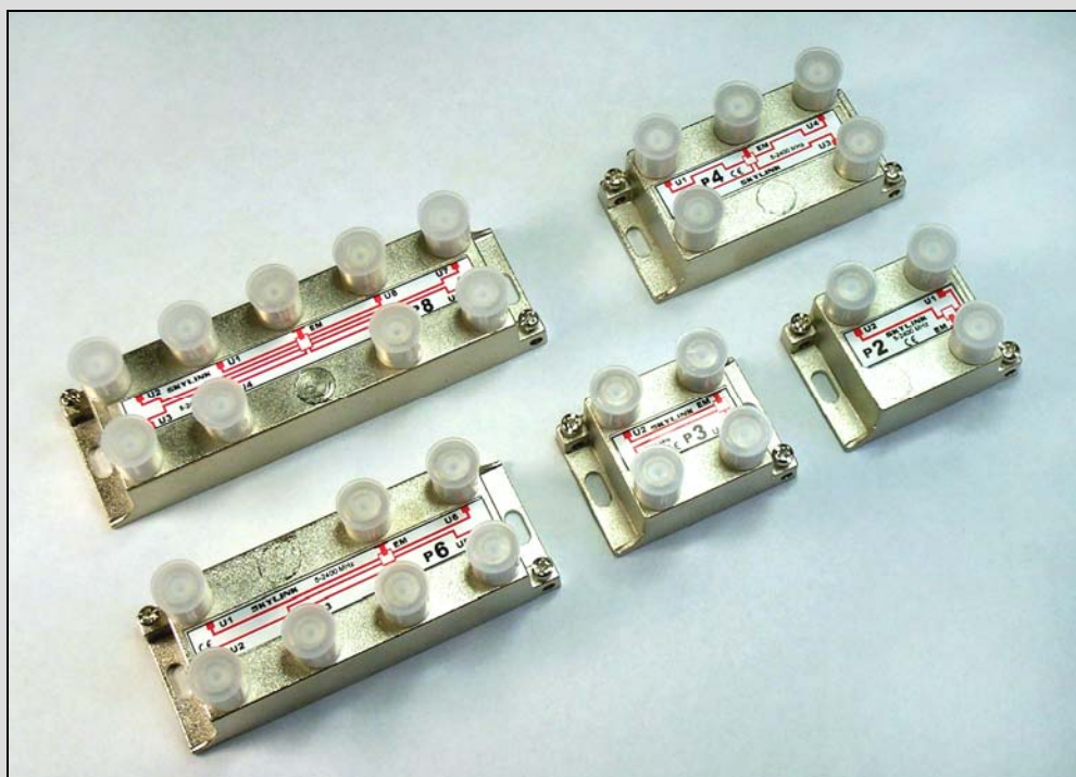
Partitori con connettori "F". Passaggio di cc su tutte le uscite.
