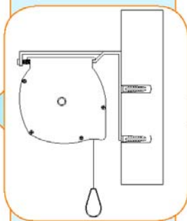
Installazione a parete
