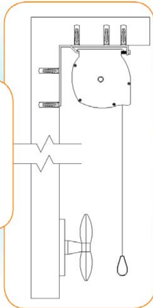
Installazione a parete
