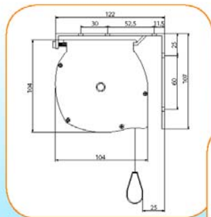
Disegni Tecnici del cassonetto Ellipse
