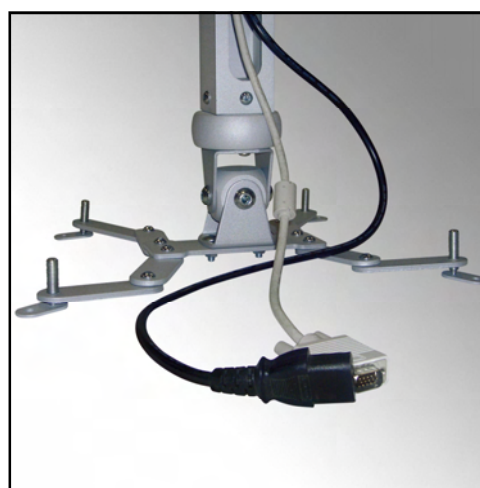
PARTICOLARE DEL PUNTO DI USCITA RISERVATO AI CAVI DEL VIDEO- PROIETTORE
