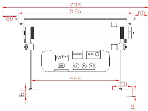
VISTA LATERALE CHIUSO
