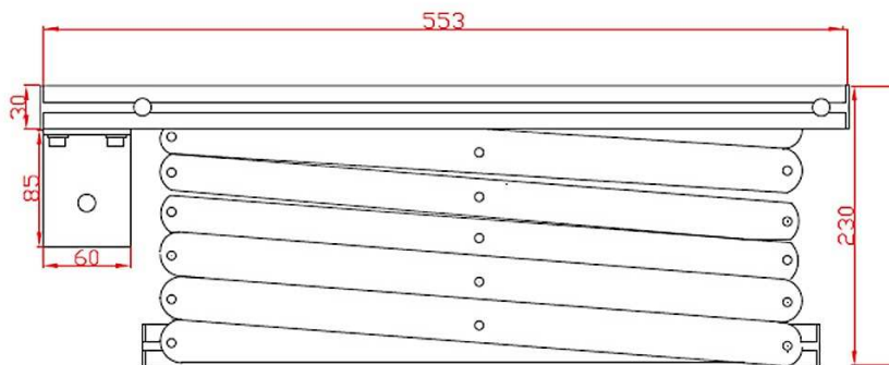
VISTA FRONTALE CHIUSO
