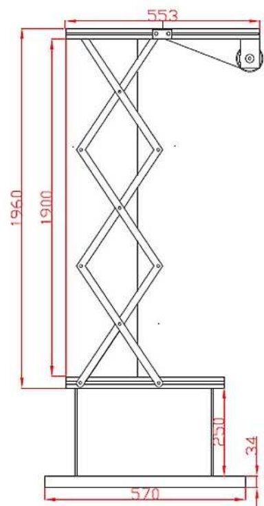
VISTA LATERALE APERTO
